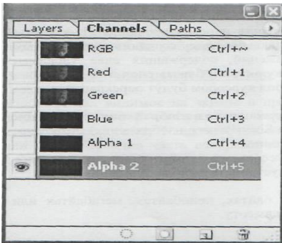
Рис. 1.4. Каналы изображения
